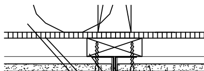
Skarvprofil 1:5
