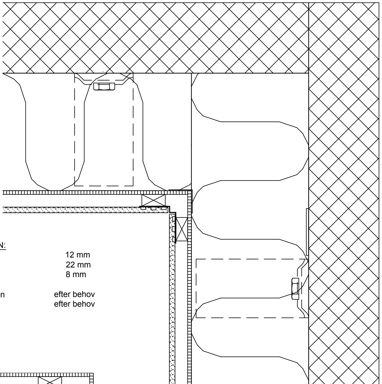
Konstruktionsprincip 2 med hörnprofil.
