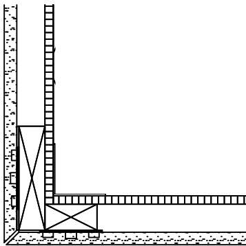
Konstruktionsprincip 1 utan profil.
