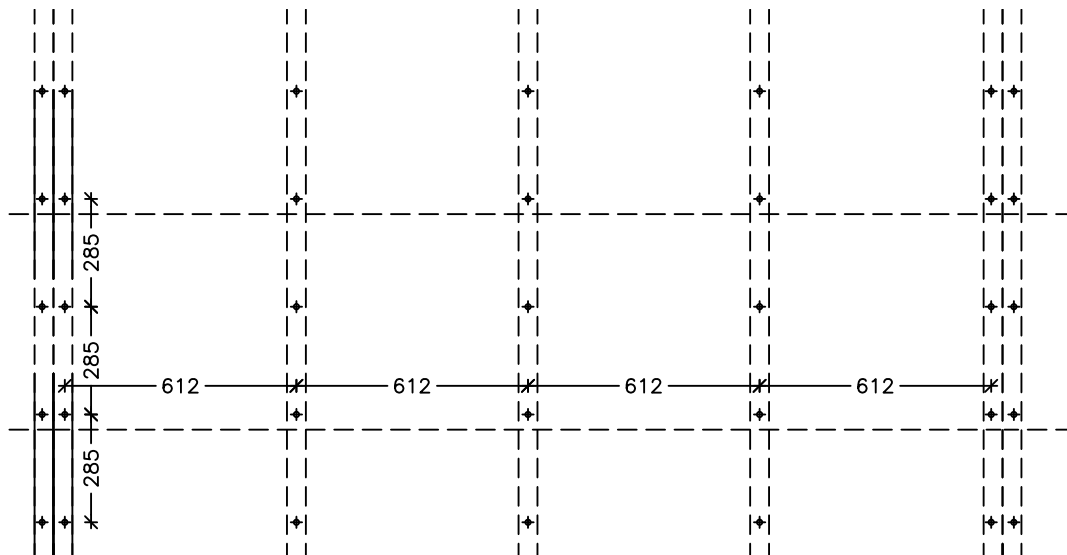
Elevation av en hel skiva 1:20
